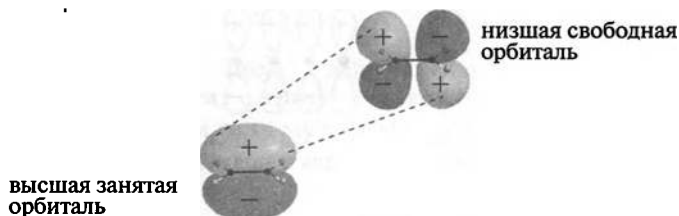
Рис. 15.3. Перекрывание орбиталей при термическом [2 + 2] -циклоприсоединении
