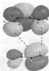
эндо , НСМО диена (сверху) перекрывается с ВЗМО акролеина (внизу)
