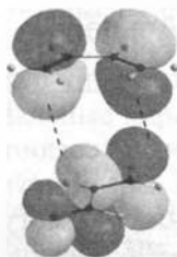
эндо , ВЗМО диена (сверху) перекрывается с НСМО акролеина (внизу)
