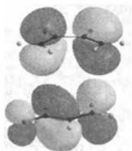
экзо , ВЗМО диена (сверху); показано плохое перекрывание с НСМО акролеина
