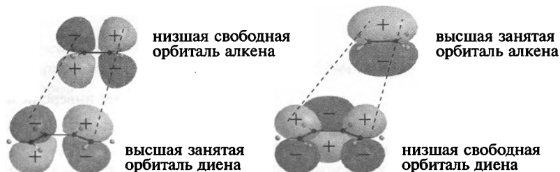
Рис. 15.4. Два пути перекрывания орбиталей при термическом [4 + 2] -циклоприсоединении
